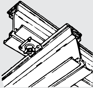
Vigueta a zanca
